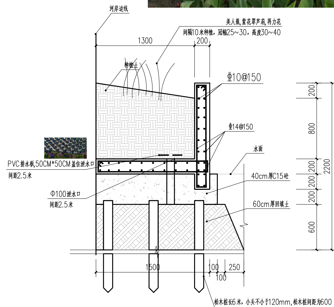
河涌南岸标准横断面设计图 1:25
