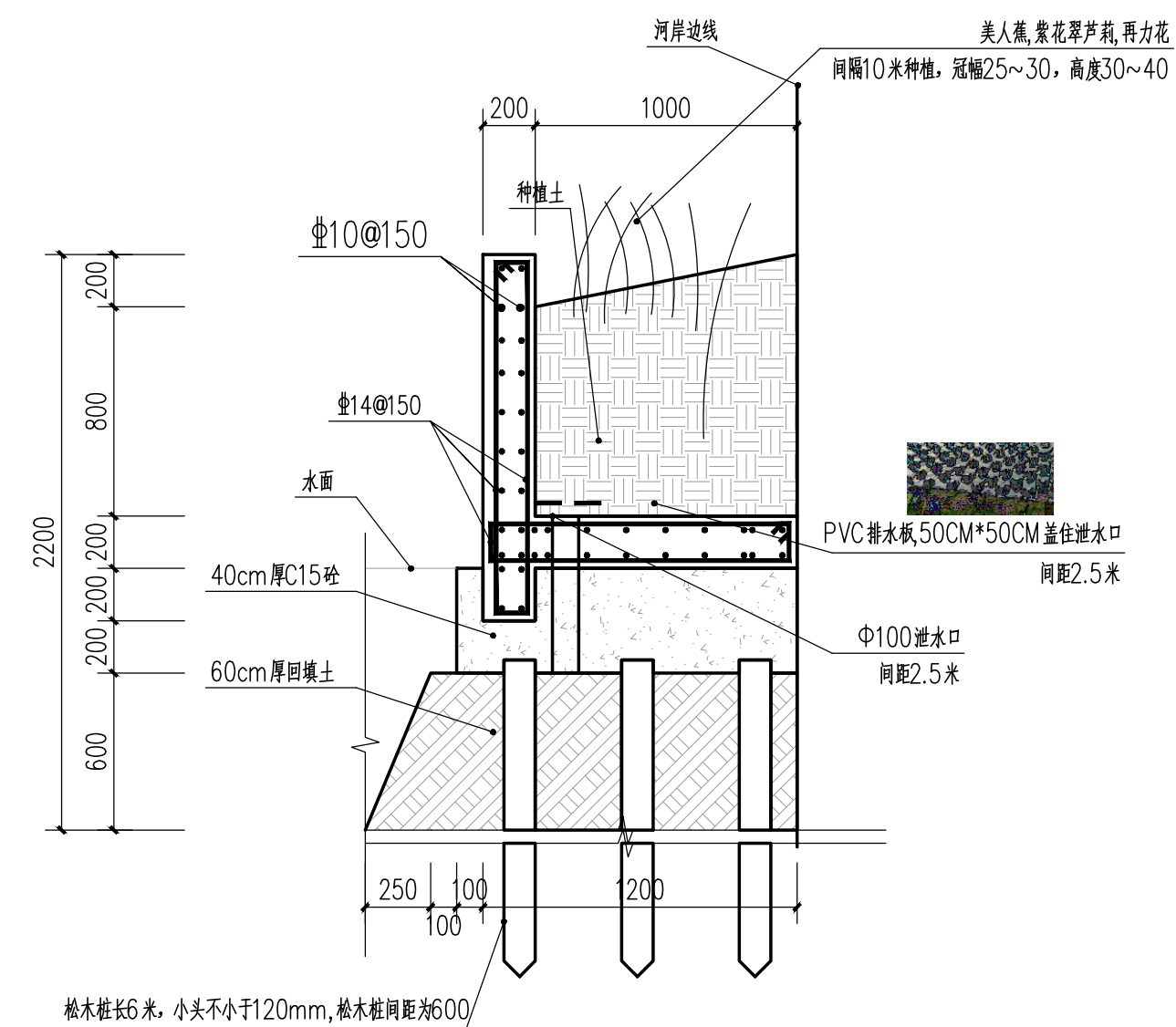
河涌北岸标准横断面设计图 1:25
